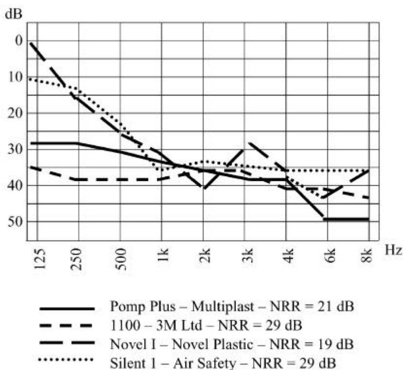
Figura 1 – Curvas de atenuação acústica média dos EPIAs usados nos ensaios.
