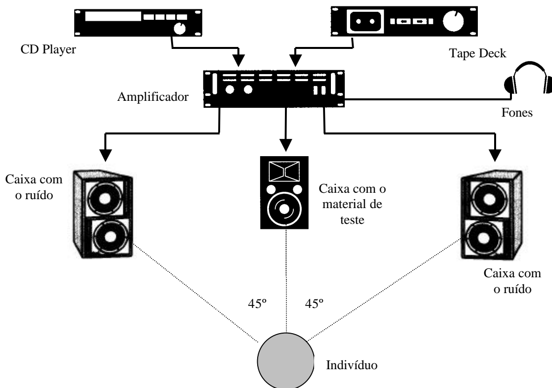
Figura 2 – Disposição dos equipamentos durante os ensaios.
