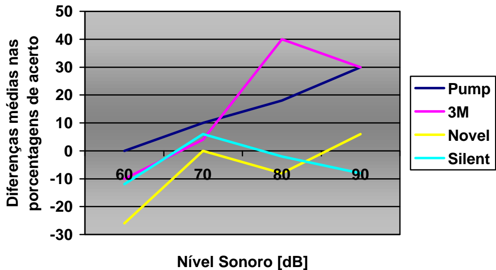
Figura 5 – Diferenças nas porcentagens de acerto (IDF) para os 4 protetores em função dos níveis sonoros.
